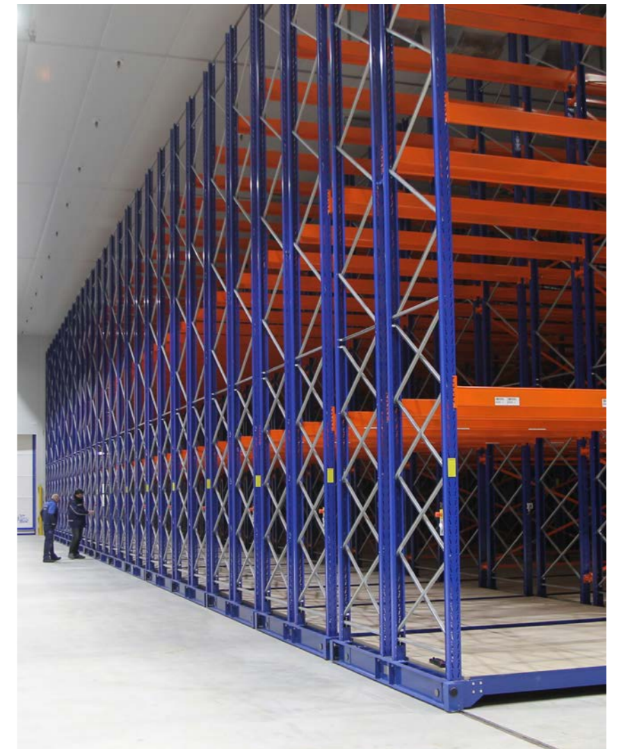
Verschieberegalen für Tiefkühlager (Leipzig)
